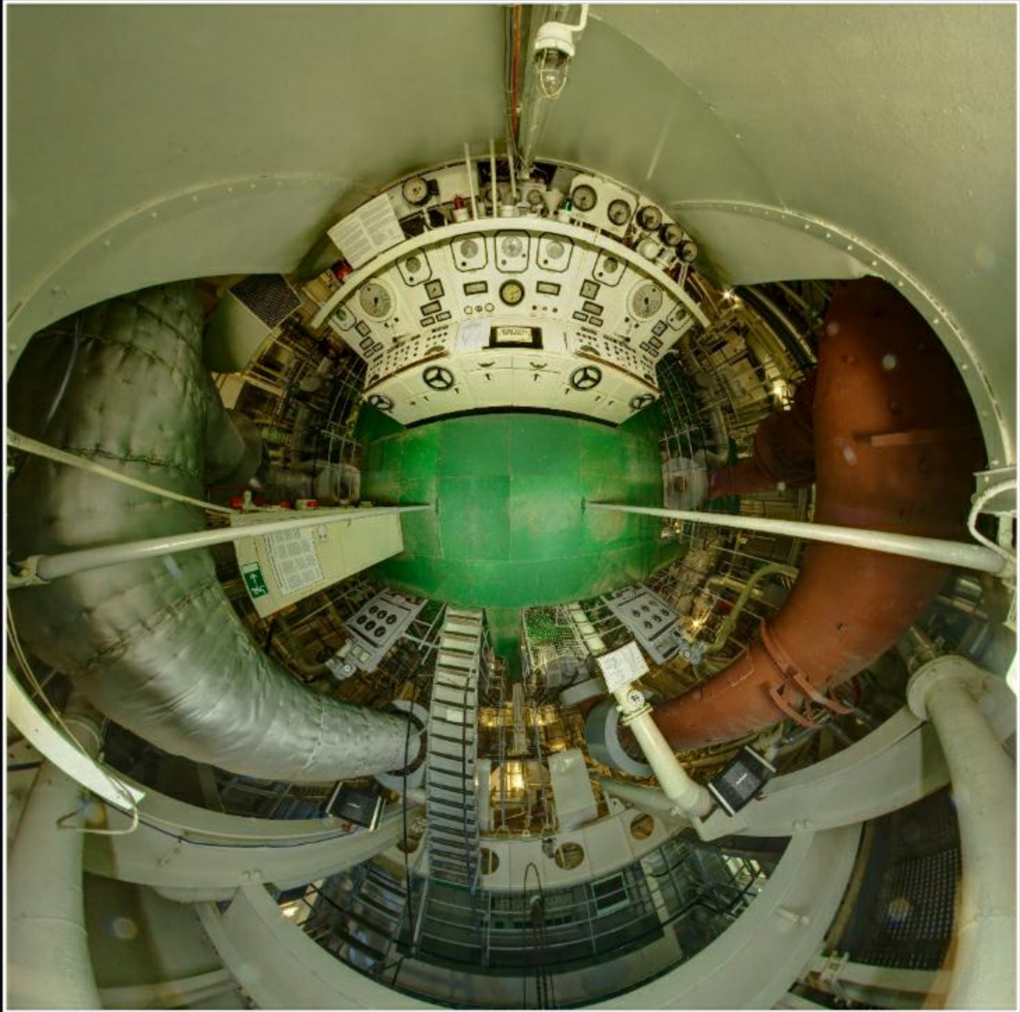
Maschinenraum, Rostocker Traditionsschiff
